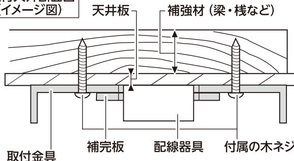
取付天井断面図 (イメージ図)
